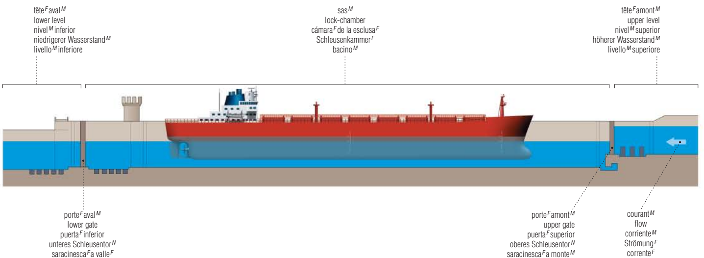
écluse F : vue F latérale canal lock: side view esclusa F : vista F lateral Kanalschleuse F : Seitenansicht F chiusa F di un canale M : vista F laterale
